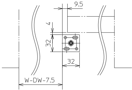
直付け下ガイド 詳細図1/4
