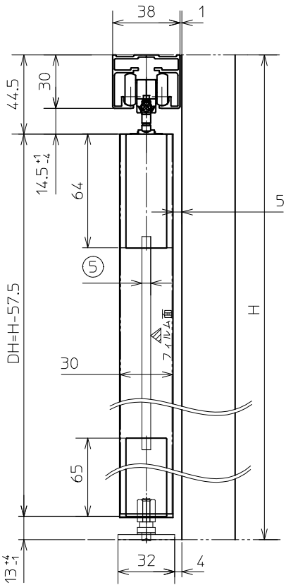
ガラス仕様 詳細図1/3
