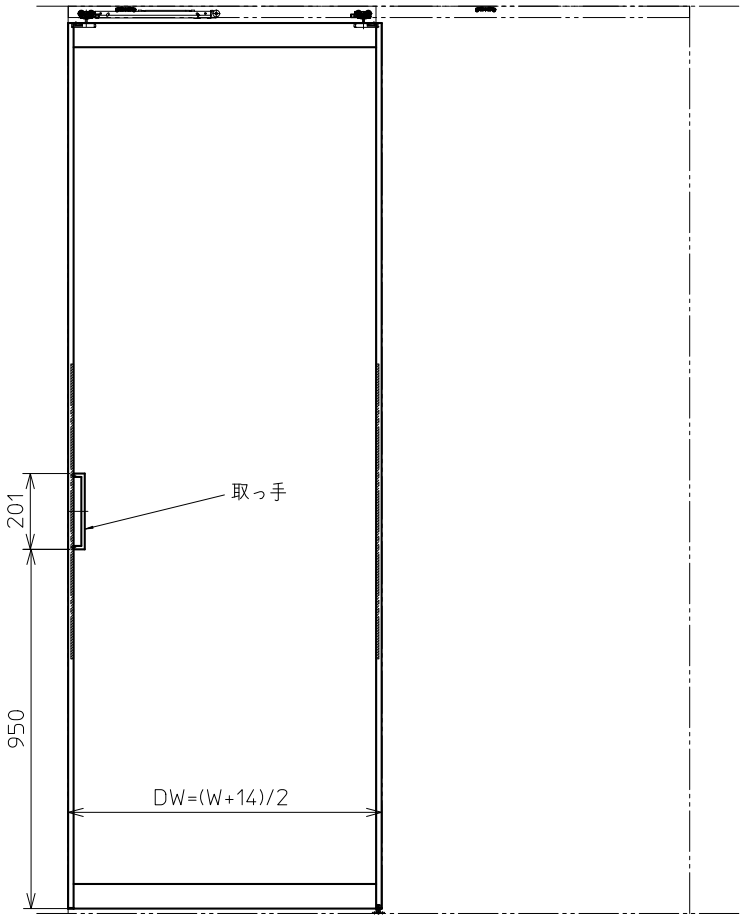
上レール直付け仕様
