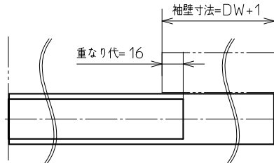
全閉時詳細図1/4
