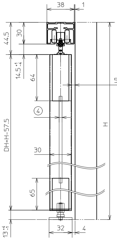
樹脂パネル仕様 詳細図1/3
