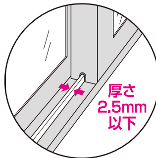
図2：下部レールがあるサッシ
