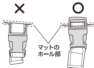
バックルの留め方（マット裏面図）
