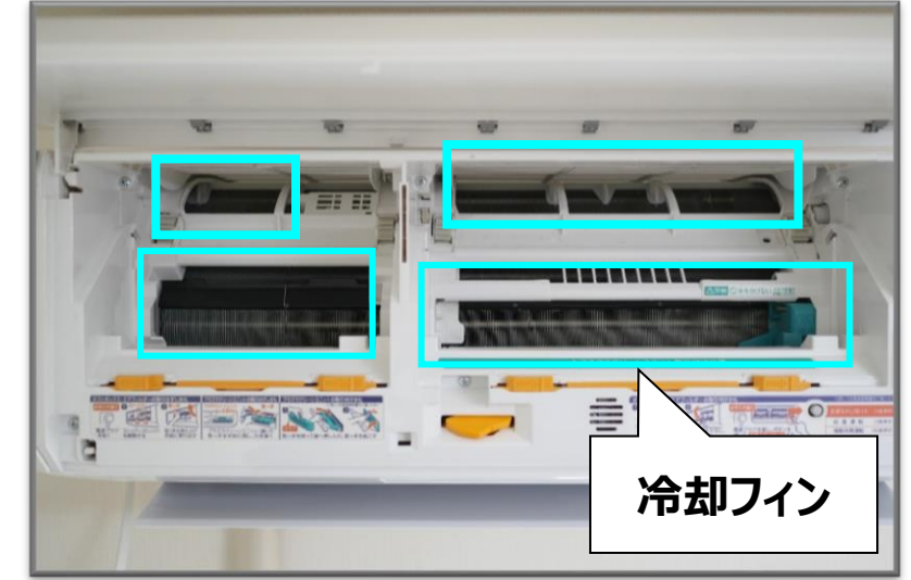
③フィルターを取り外し、フィンを露出させます。
