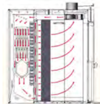
→ 熱風の流れ
