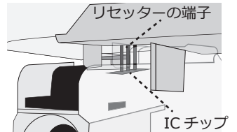
IC チップと端子の接触イメージ
