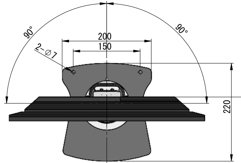
スイベル可動範囲
