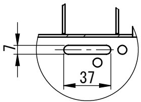
詳細図 B スケール 1 : 3
