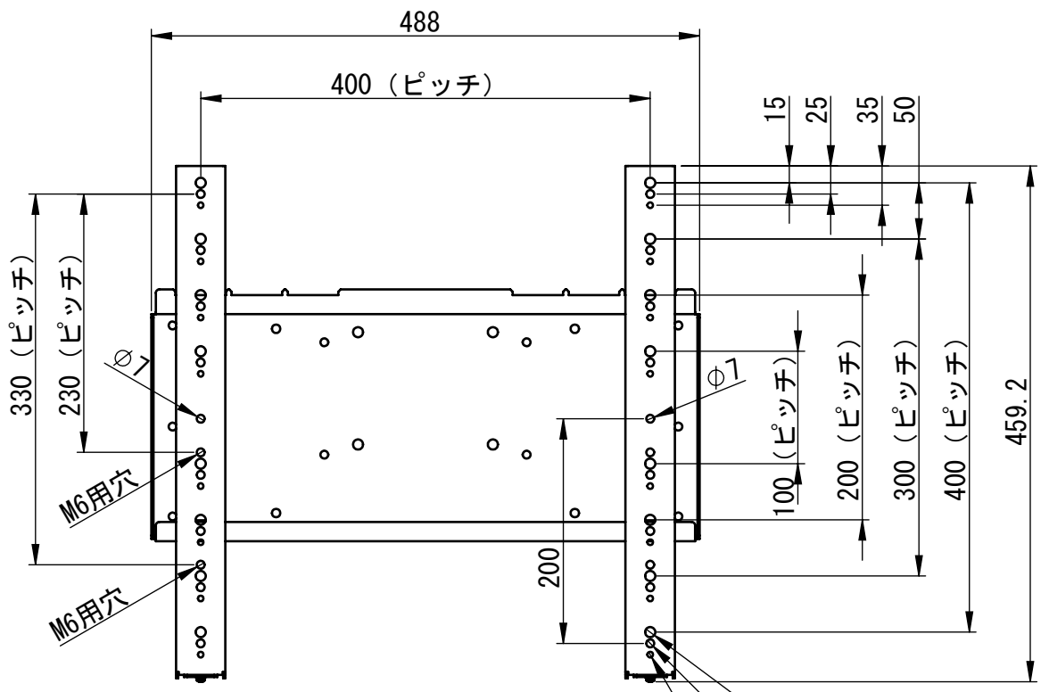
400mmピッチレイアウト
