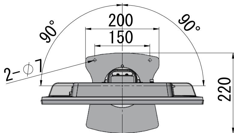
スイベル可動範囲 443
