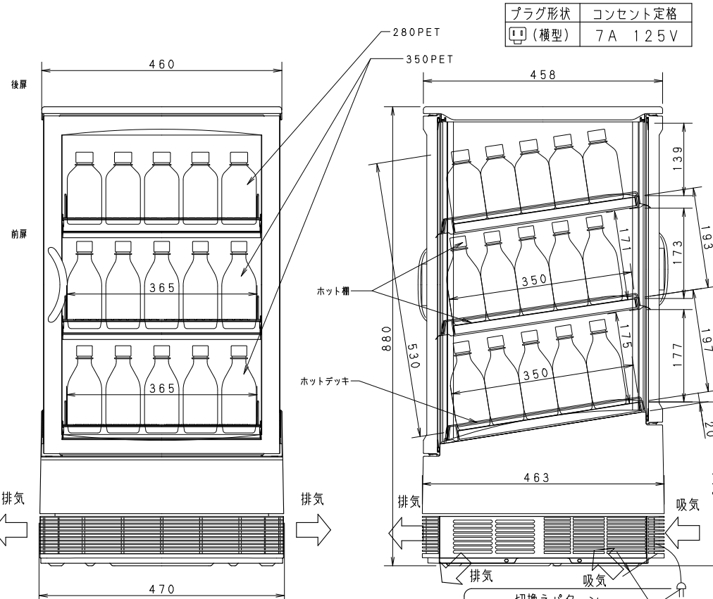
350ml PETボトル収容図
