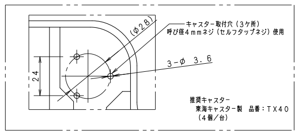
キャスター取付用 参考寸法図
