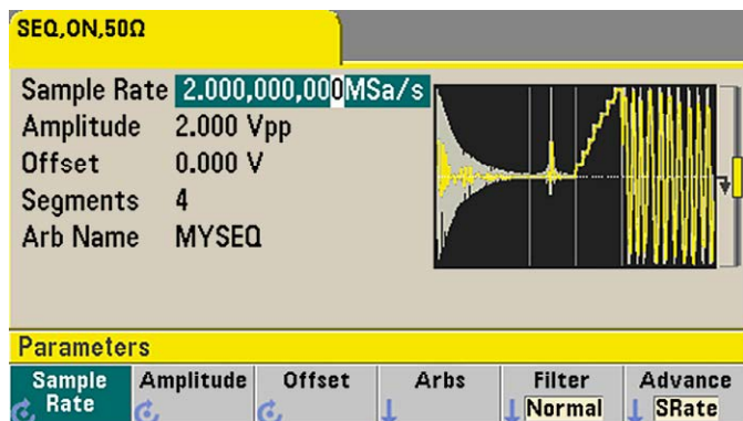
必要なシーケンスが表示された波形発生器のディスプレイ。
