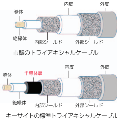
キーサイトの標準トライアキシャルケーブル
