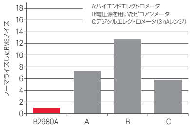
2 nAレンジのRMSノイズ（ノーマライズ後） 0.1 PLC、3 mトライアキシャルケーブルを使用
