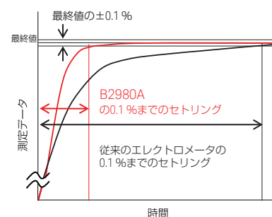
20 pAレンジのセトリング時間 2 Vステップ、100 GΩ、1 PLC
