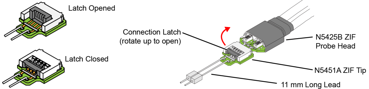
Figure 49 N5451A ZIF Tip Trimmed to 11 mm
