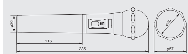
外形寸法図 [WM-P970/P902] (単位:mm)
