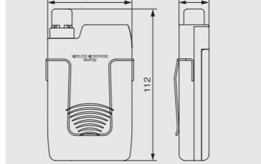
外形寸法図 [WM-P980] (単位:mm)
