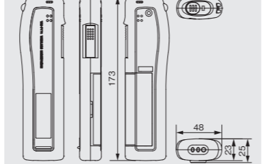
外形寸法図 [WM-P772] (単位:mm)
