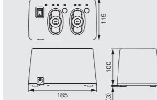
外形寸法図 (単位:mm)
