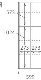
正面図
