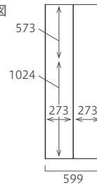
正面図
