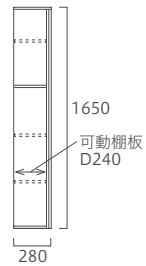
側面図
