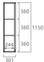
側面図
