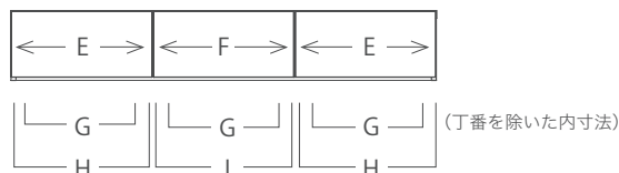
正面図
