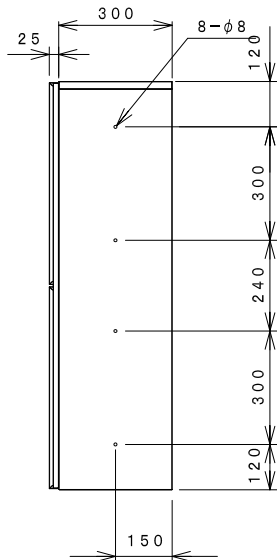
側面図
