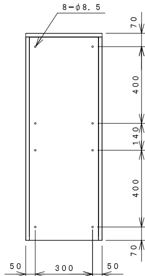
背面図
