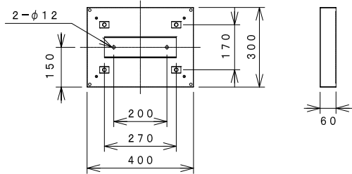
TBX-H(HS) 幅木
