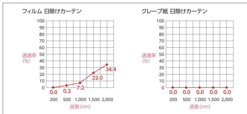
日除けカーテン透過率比較実験
