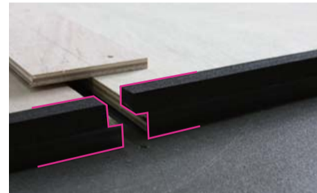
交互に重なる様に貼れば収まりがキレイになります
