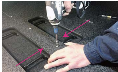
接合部分の板と板をしっかり寄せながら 3x20mm のビスで固定して下さい
