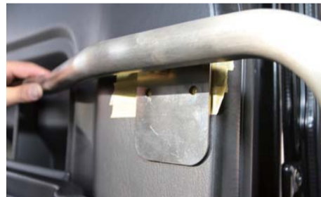
助手席側フレームを仮固定し、干渉部分にマスキングテープ等で穴位置をマークする
