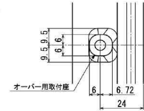
A ダッチインサート取付部詳細
