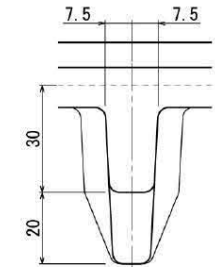
A ダッチインサート取付部詳細
