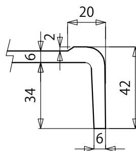
B-B断面図 S≒1:2
