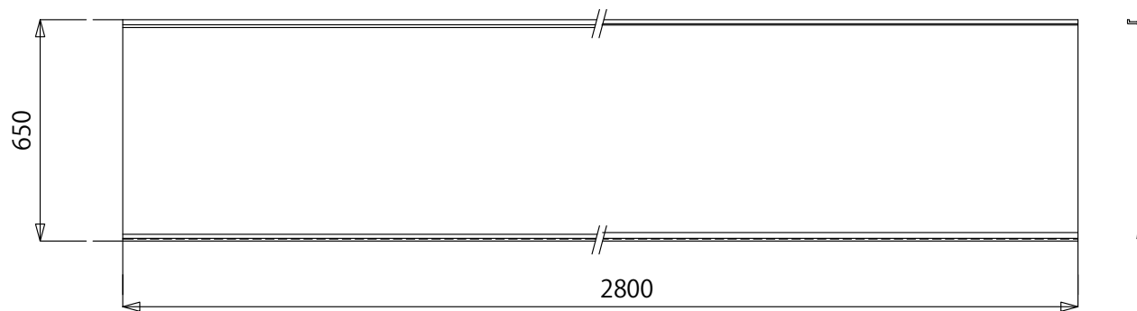
平面図 S≒1:20
