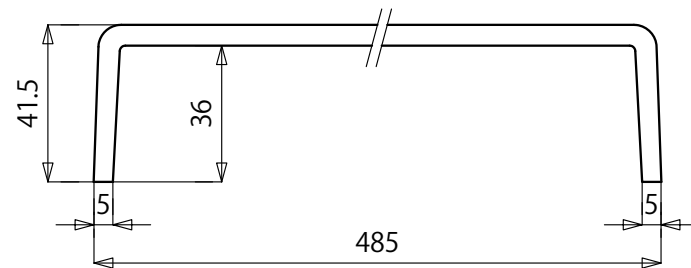
A-A断面図 S≒1:2
