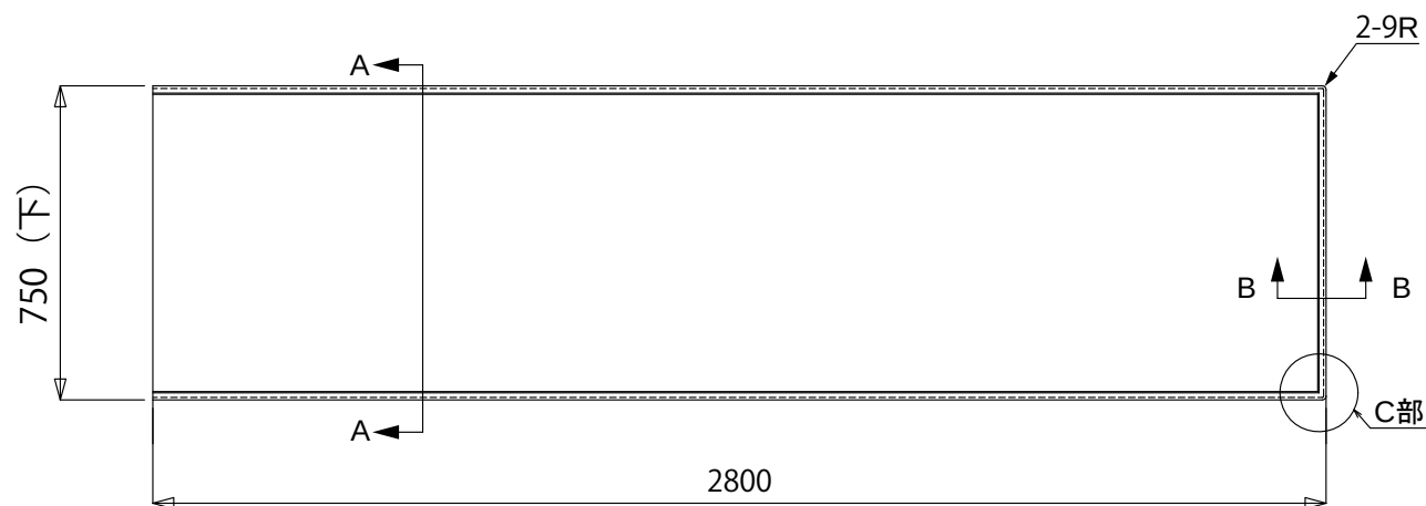
平面図 S≒1:20
