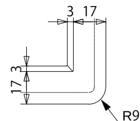
C部詳細図 S≒1:2
