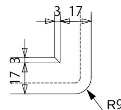
C部詳細図 S≒1:2
