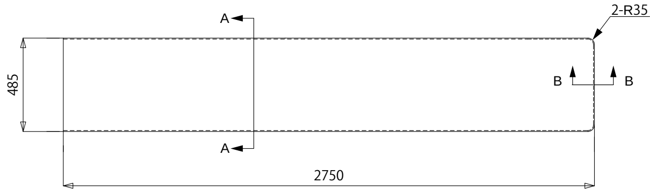
平面図 S≒1:20
