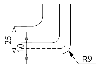
C部詳細図 S≒1:2
