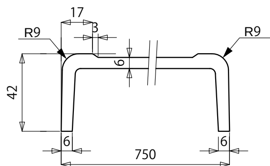
A-A断面図 S≒1:2
