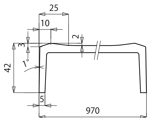
A-A断面図 S≒1:2
