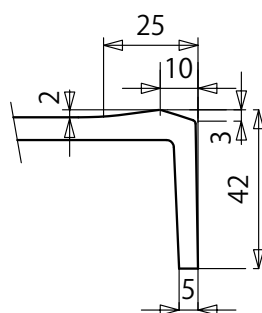
B-B断面図 S≒1:2
