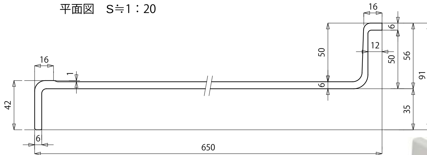
断面図 S≒1:2
