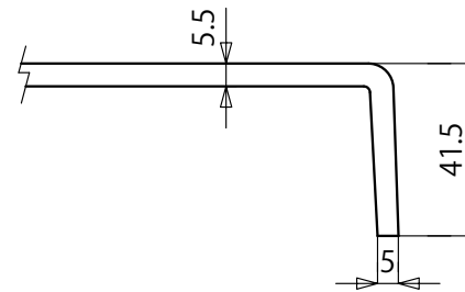
B-B断面図 S≒1:2
