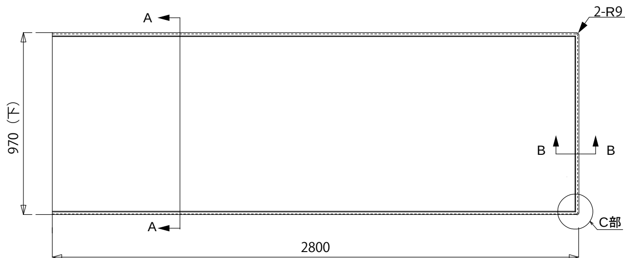
平面図 S≒1:20
