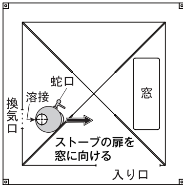
ストーブ配置平面図
