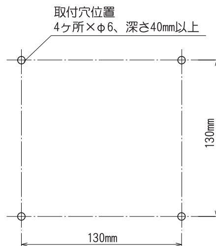
穴加工図
