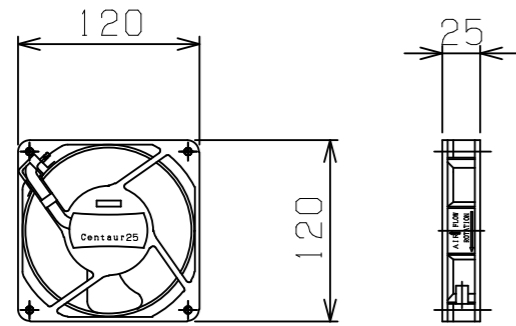
オプションファン寸法
