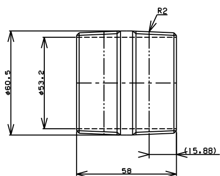
TITLE ニップル MODEL R-7G-2
