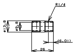
TITLE ニップル MODEL R-7G-1/4
