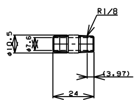
TITLE ニップル MODEL R-7G-1/8
