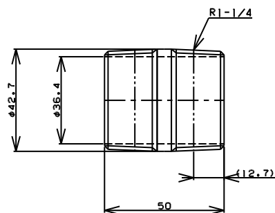
TITLE ニップル MODEL R-7G-1-1/4
