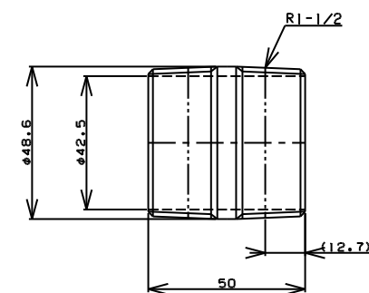
TITLE ニップル MODEL R-7G-1-1/2
