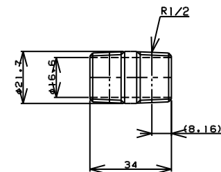
TITLE ニップル MODEL R-7G-1/2
