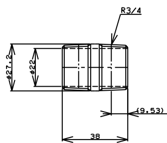
TITLE ニップル MODEL R-7G-3/4
