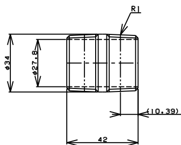
TITLE 片ニップル MODEL R-7G-1
