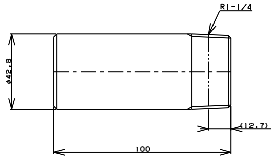
TITLE 片長ニップル MODEL R-7F-1-1/4 L=100
