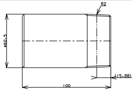
TITLE 片長ニップル MODEL R-7F-2 L=100
