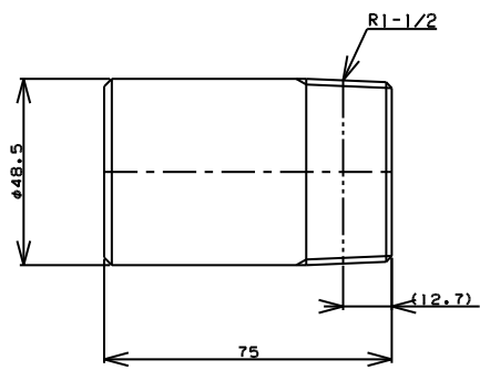
TITLE 片長ニップル MODEL R-7F-1-1/2 L=75
