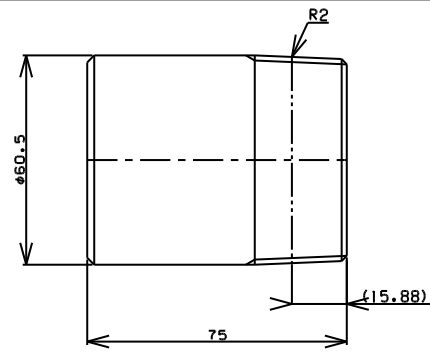
TITLE 片長ニップル MODEL R-7F-2 L=75
