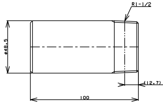
TITLE 片長ニップル MODEL R-7F-1-1/2 L=100
