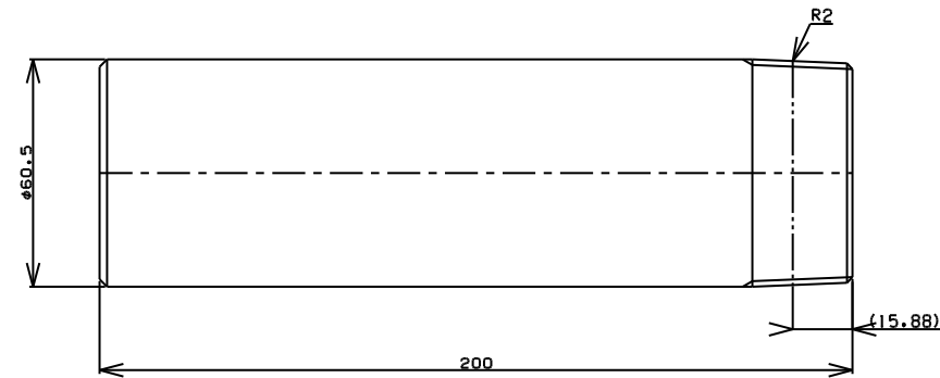
TITLE 片長ニップル MODEL R-7F-2 L=200
