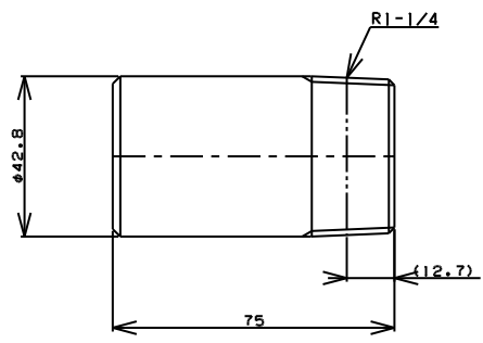
TITLE 片長ニップル MODEL R-7F-1-1/4 L=75
