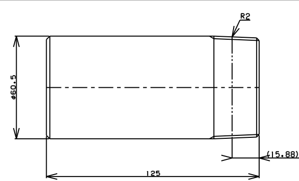
TITLE 片長ニップル MODEL R-7F-2 L=125
