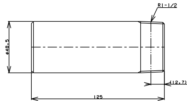
TITLE 片長ニップル MODEL R-7F-1-1/2 L=125
