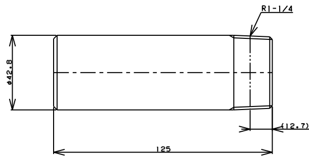
TITLE 片長ニップル MODEL R-7F-1-1/4 L=125
