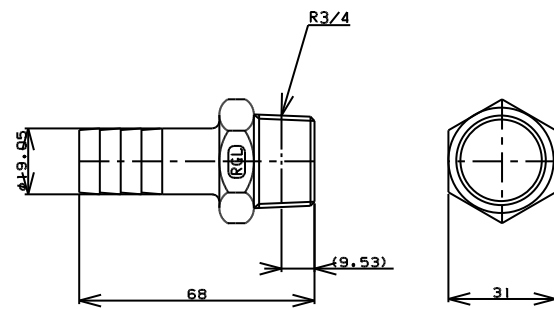
TITLE ホースニップル MODEL R-7D-3/4
