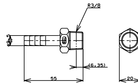
TITLE ホースニップル MODEL R-7D-3/8
