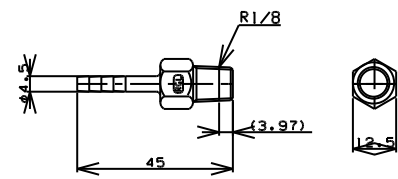
TITLE ホースニップル MODEL R-7D-1/8
