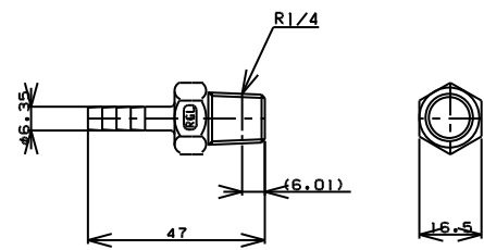
TITLE ホースニップル MODEL R-7D-1/4
