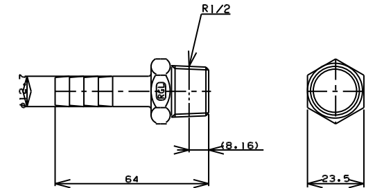
TITLE ホースニップル MODEL R-7D-1/2
