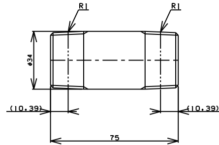
TITLE 両長ニップル MODEL R-7B-1 L=75
