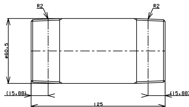
TITLE 両長ニップル MODEL R-7B-2 L=125
