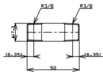
TITLE 両長ニップル MODEL R-7B-3/8 L=50
