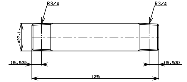
TITLE 両長ニップル MODEL R-7B-3/4 L=125
