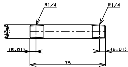
TITLE 両長ニップル MODEL R-7B-1/4 L=75
