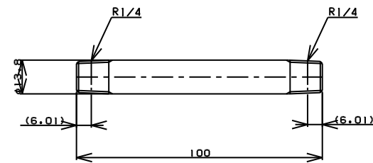
TITLE 両長ニップル MODEL R-7B-1/4 L=100
