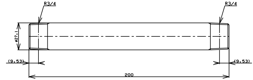
TITLE 両長ニップル MODEL R-7B-3/4 L=200
