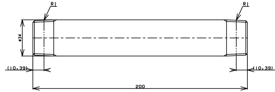
TITLE 両長ニップル MODEL R-7B-1 L=200
