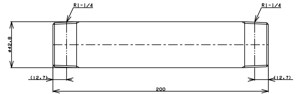
TITLE 両長ニップル MODEL R-7B-1-1/4 L=200
