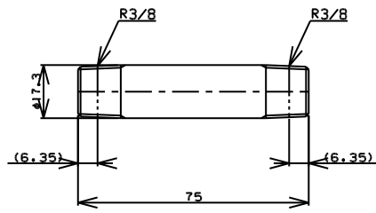
TITLE 両長ニップル MODEL R-7B-3/8 L=75
