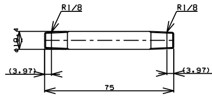
TITLE 両長ニップル MODEL R-7B-1/8 L=75
