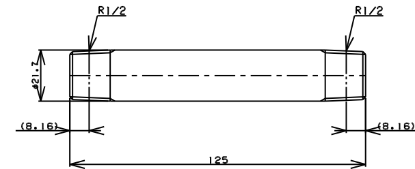
TITLE 両長ニップル MODEL R-7B-1/2 L=125
