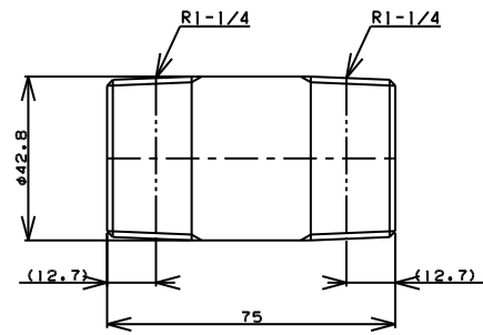
TITLE 両長ニップル MODEL R-7B-1-1/4 L=75
