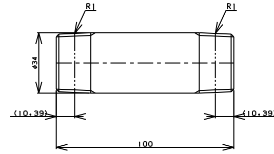
TITLE 両長ニップル MODEL R-7B-1 L=100
