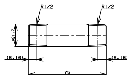
TITLE 両長ニップル MODEL R-7B-1/2 L=75
