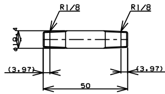
TITLE 両長ニップル MODEL R-7B-1/8 L=50
