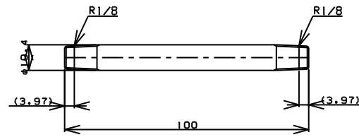
TITLE 両長ニップル MODEL R-7B-1/8 L=100
