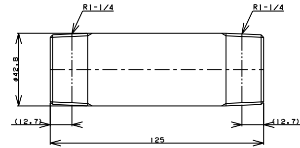
TITLE 両長ニップル MODEL R-7B-1-1/4 L=125
