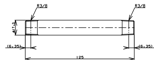
TITLE 両長ニップル MODEL R-7B-3/8 L=125
