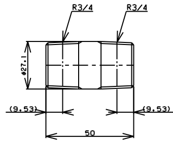
TITLE 両長ニップル MODEL R-7B-3/4 L=50
