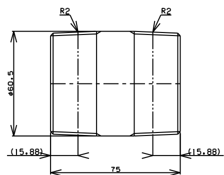
TITLE 両長ニップル MODEL R-7B-2 L=75
