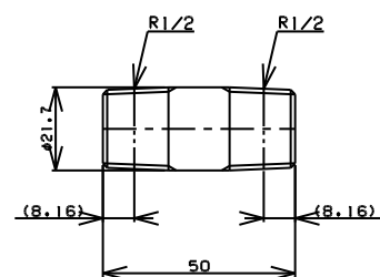
TITLE 両長ニップル MODEL R-7B-1/2 L=50
