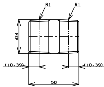
TITLE 両長ニップル MODEL R-7B-1 L=50
