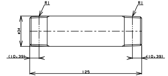
TITLE 両長ニップル MODEL R-7B-1 L=125
