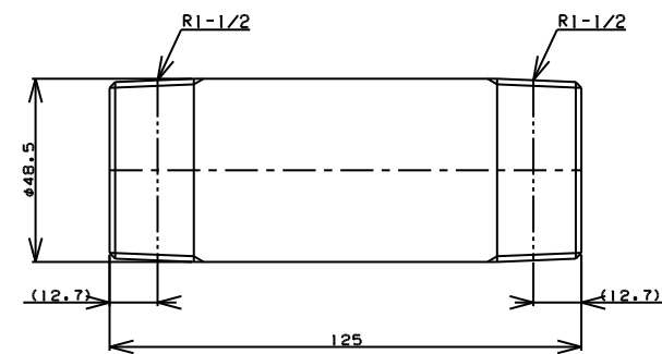
TITLE 両長ニップル MODEL R-7B-1-1/2 L=125
