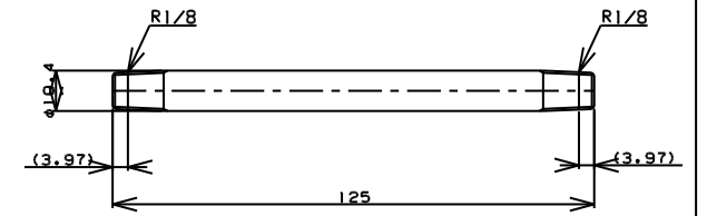
TITLE 両長ニップル MODEL R-7B-1/8 L=125
