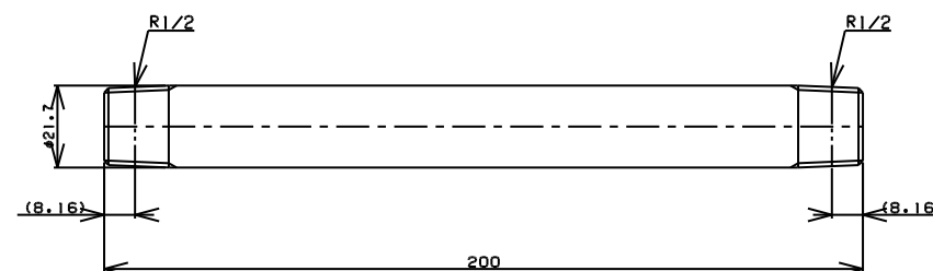
TITLE 両長ニップル MODEL R-7B-1/2 L=200
