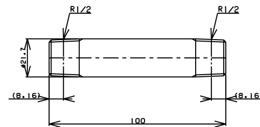
TITLE 両長ニップル MODEL R-7B-1/2 L=100
