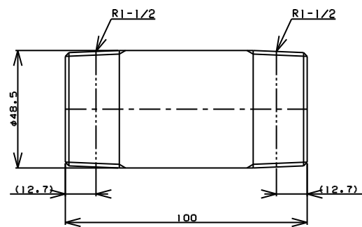
TITLE 両長ニップル MODEL R-7B-1-1/2 L=100
