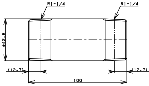
TITLE 両長ニップル MODEL R-7B-1-1/4 L=100
