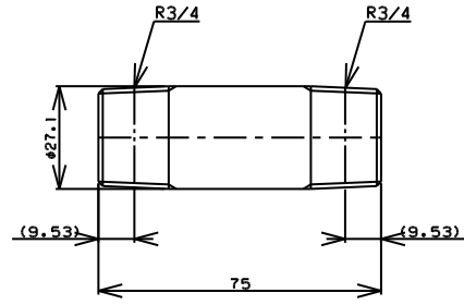
TITLE 両長ニップル MODEL R-7B-3/4 L=75
