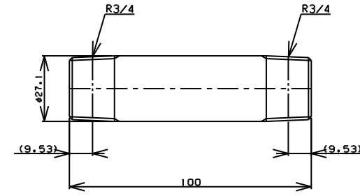
TITLE 両長ニップル MODEL R-7B-3/4 L=100
