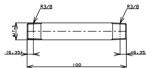
TITLE 両長ニップル MODEL R-7B-3/8 L=100
