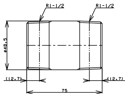
TITLE 両長ニップル MODEL R-7B-1-1/2 L=75
