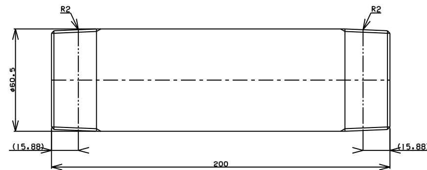
TITLE 両長ニップル MODEL R-7B-2 L=200
