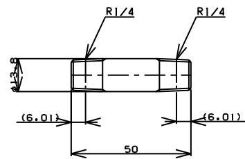
TITLE 両長ニップル MODEL R-7B-1/4 L=50
