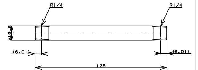
TITLE 両長ニップル MODEL R-7B-1/4 L=125
