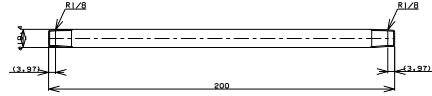
TITLE 両長ニップル MODEL R-7B-1/8 L=200
