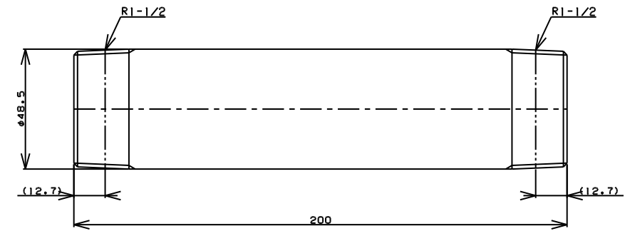
TITLE 両長ニップル MODEL R-7B-1-1/2 L=200
