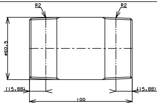
TITLE 両長ニップル MODEL R-7B-2 L=100
