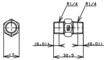
TITLE 六角ニップル MODEL R-72-1/4
