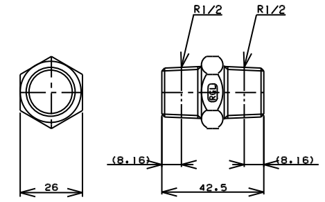
TITLE 六角ニップル MODEL R-72-1/2
