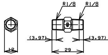
TITLE 六角ニップル MODEL R-72-1/8
