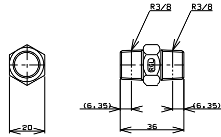
TITLE 六角ニップル MODEL R-72-3/8
