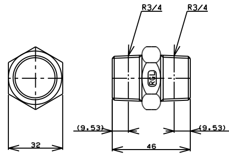
TITLE 六角ニップル MODEL R-72-3/4
