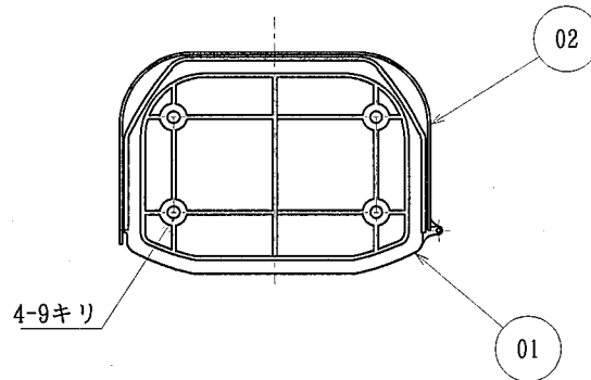
底部詳細図
