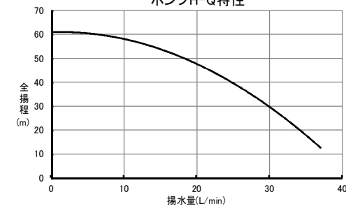
ポンプH-Q特性
