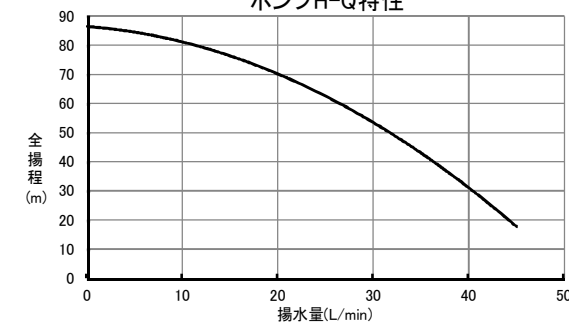
ポンプH-Q特性
