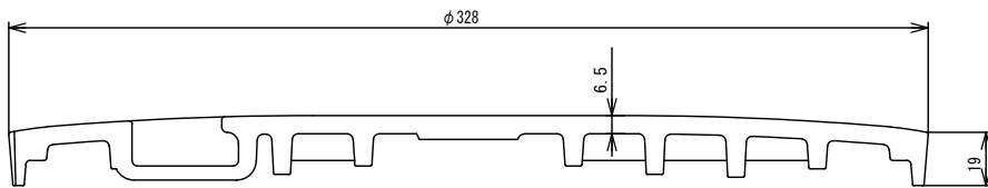
A-A' 断面図
