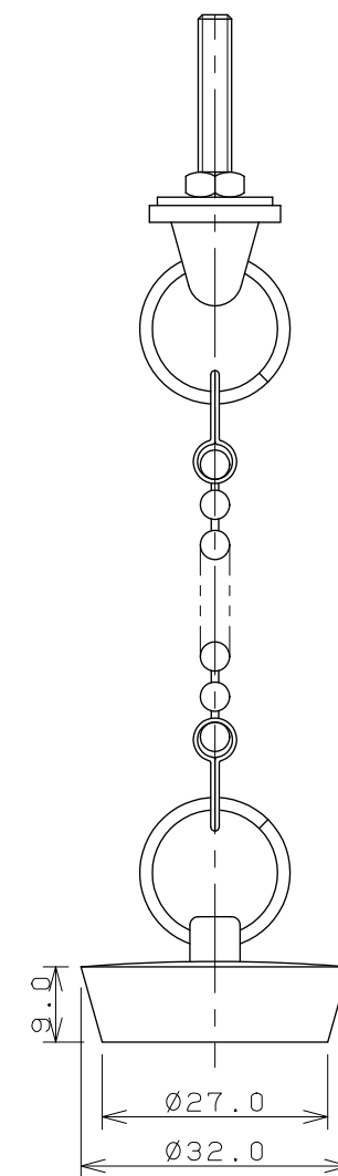
ゴム栓 (1/1)
