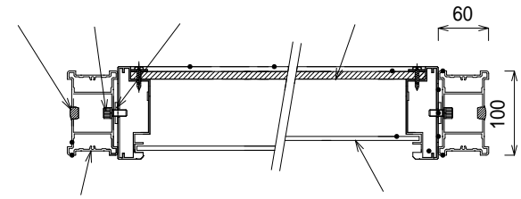
断面 B - B (S = 1 / 6)
