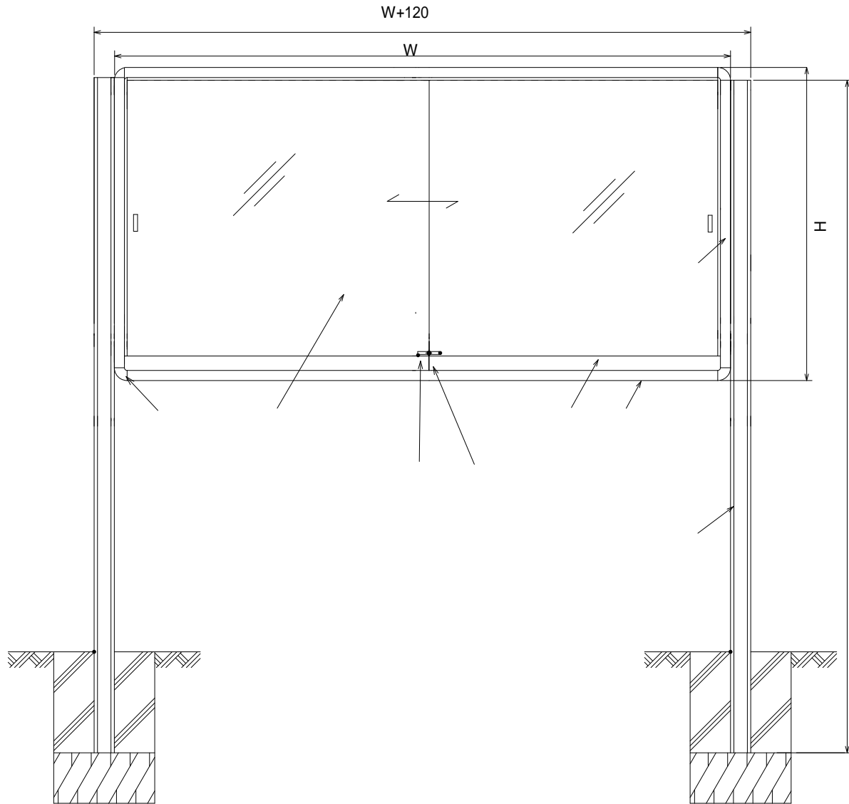
支柱横付タイプ
