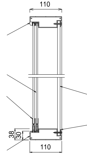
断面 A - A (S = 1 / 6)
