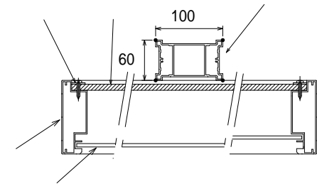
断面 B - B (S = 1 / 6)
