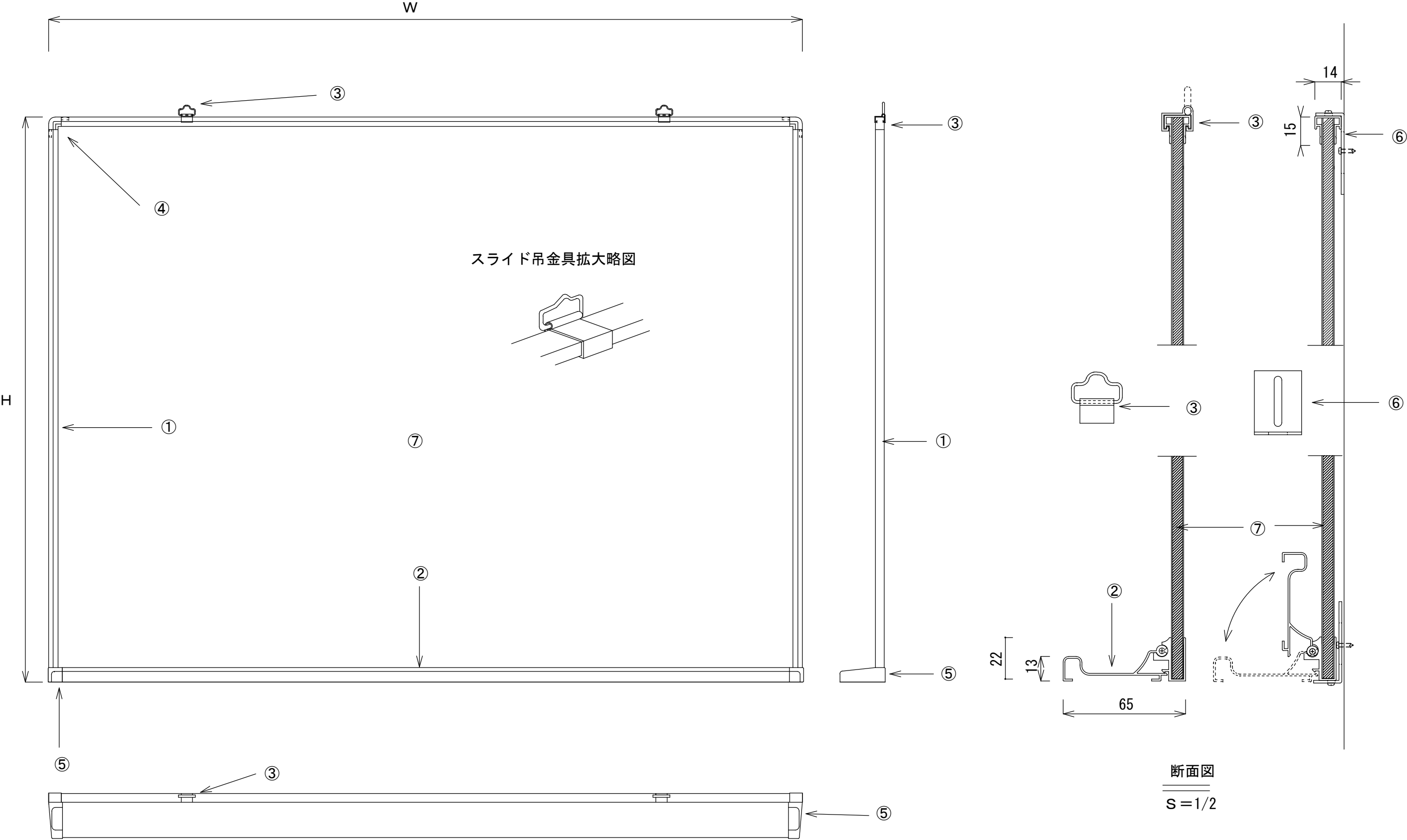
正面図 A3 S=1/6
