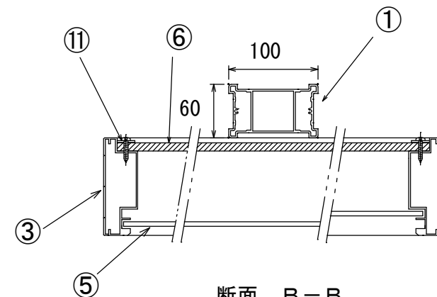
断面 B-B (S=1/6)
