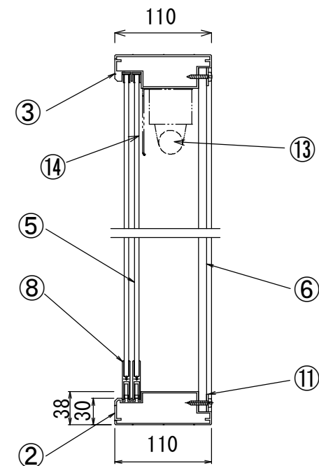
断面 A-A (S=1/6)
